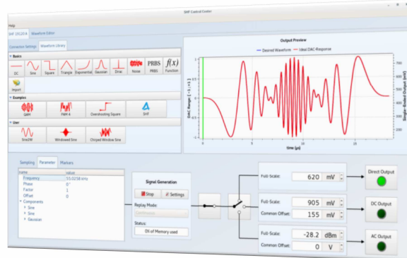
SHF 19120 B: actual waveform and GUI
